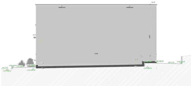
Südwestfassade
