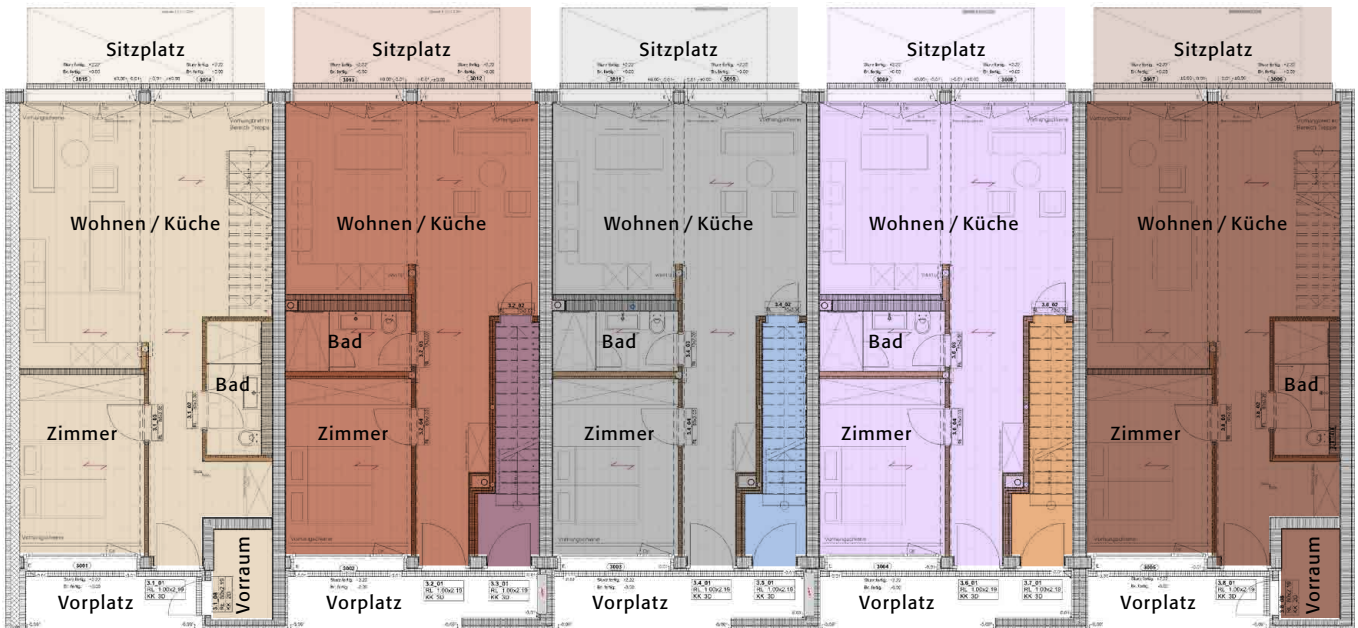
Erdgeschoss
