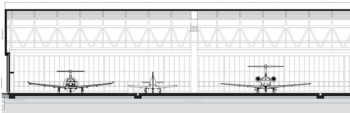
Schnitt D
