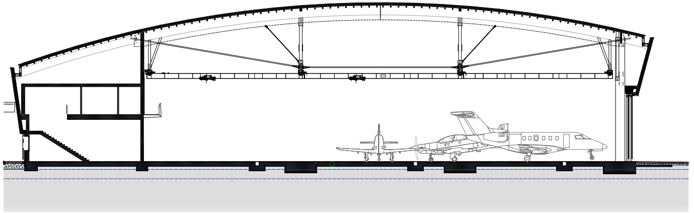
Schnitt A
