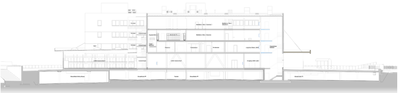
Südschnitt
