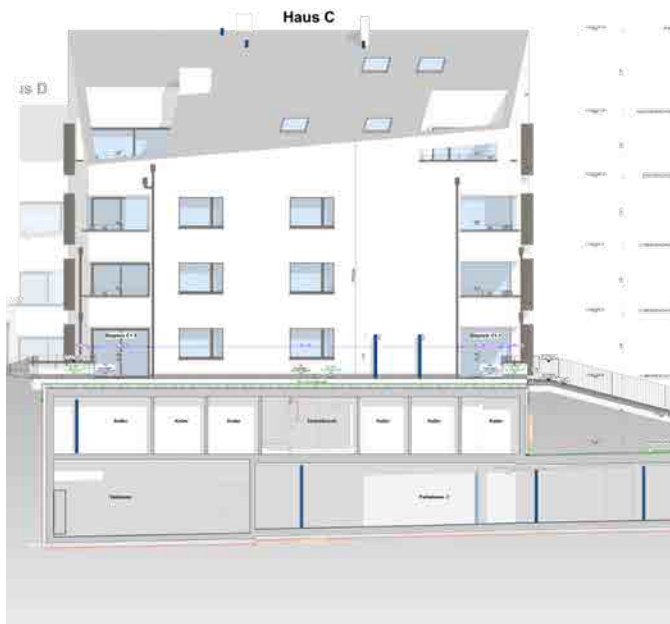
Südfassade
