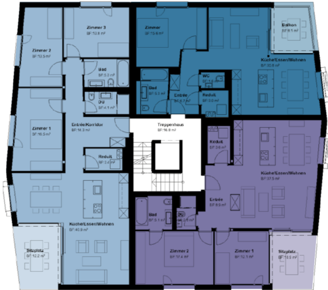
Erdgeschoss
