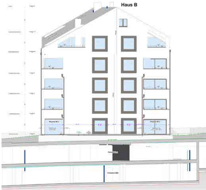
Südfassade
